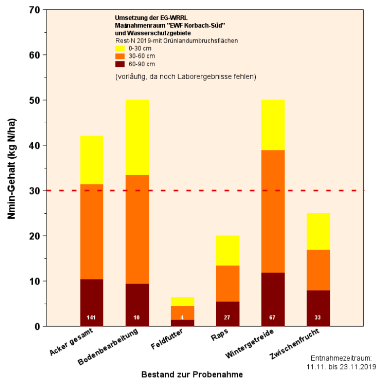
Abb. 1: Mittlere Rest-N-Gehalte der Bodenschichten im Maßnahmenraum EWF Korbach-Süd nach Begrünung
